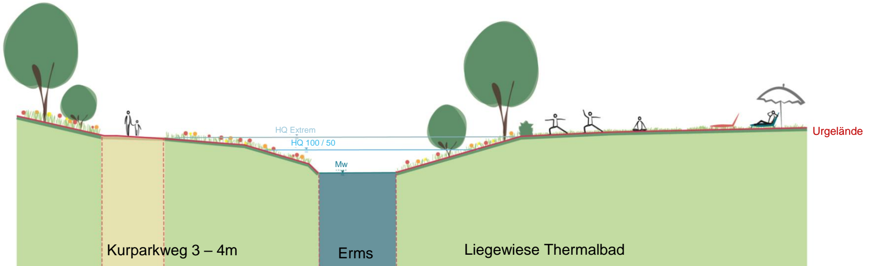
Schnitt 4 Kurpark - Albthermen
