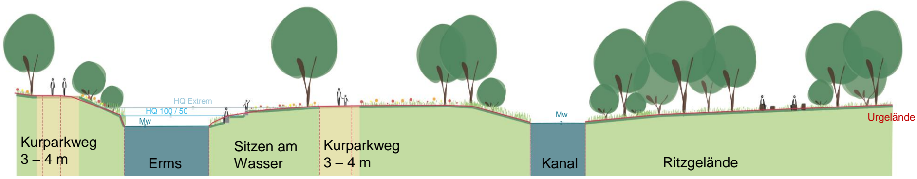
Schnitt 6a Kurpark - Kanal
