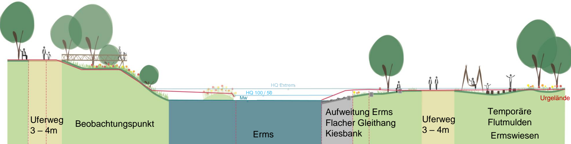
Schnitt 8 Ermswiesen – alter Kanal
