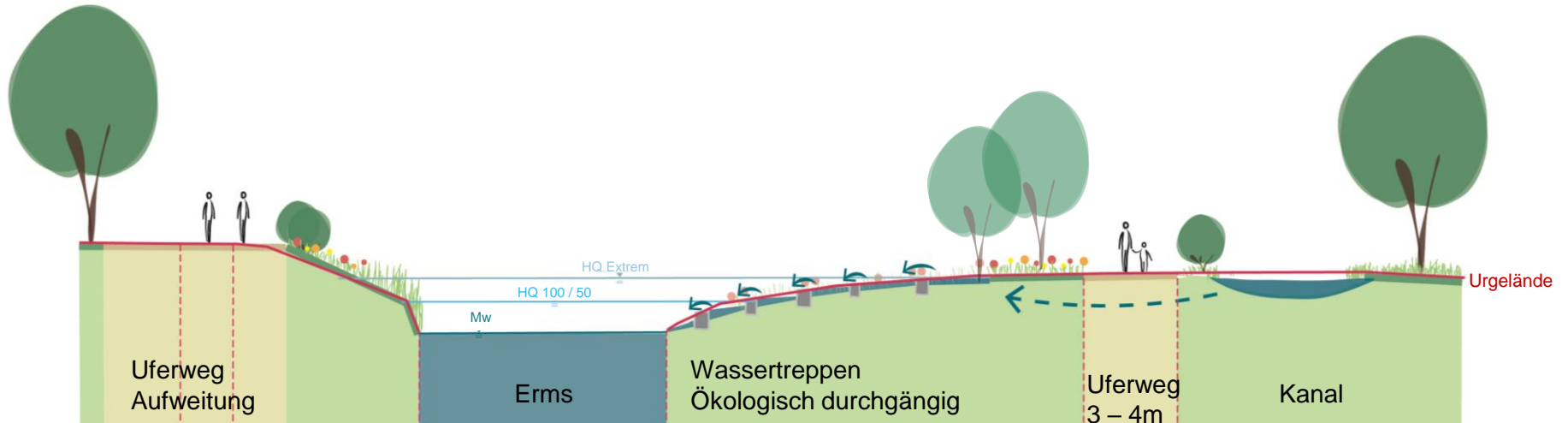
Schnitt 6b Kurpark - Wasserkaskaden Erms
