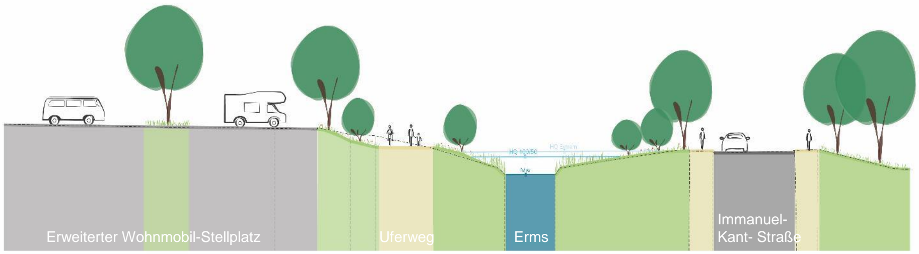
Schnitt 2 Wohnmobil-Stellplatz
