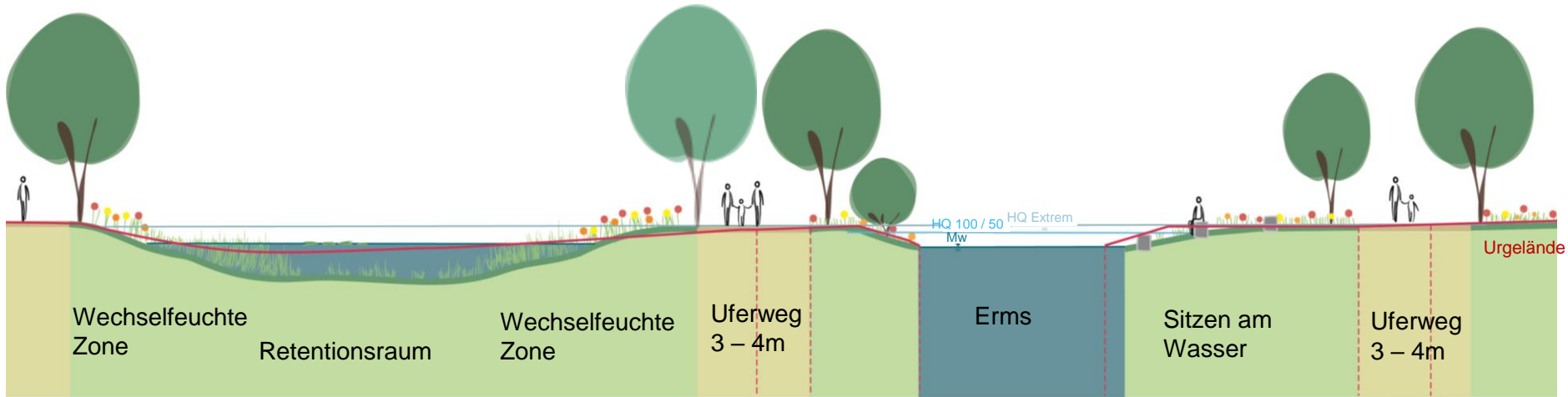
Schnitt 10a Ermswiesen – Retentionsraum
